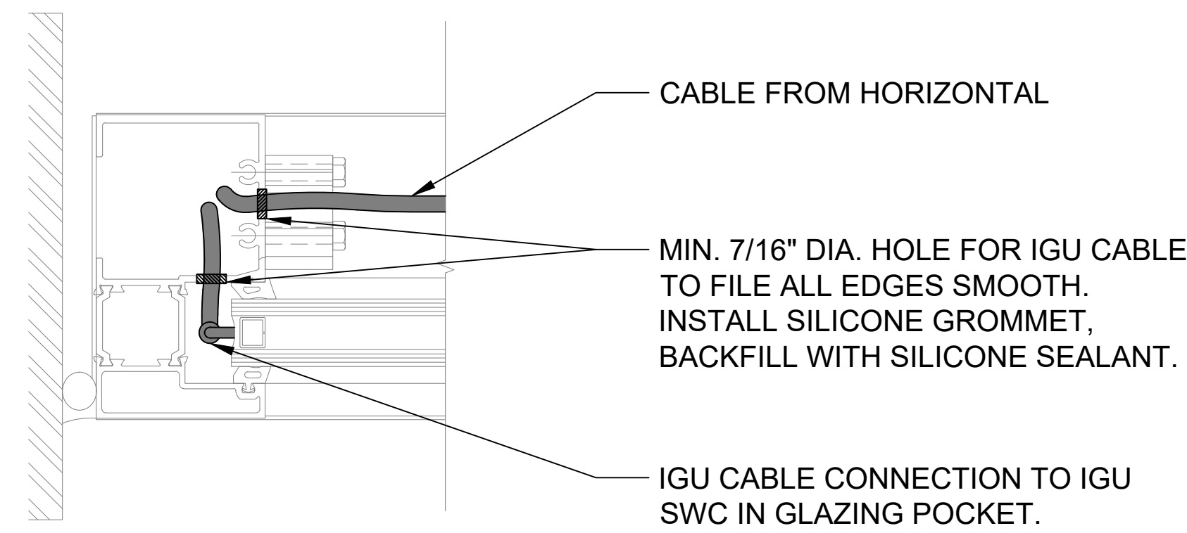
DETAIL 4 LEFT JAMB
